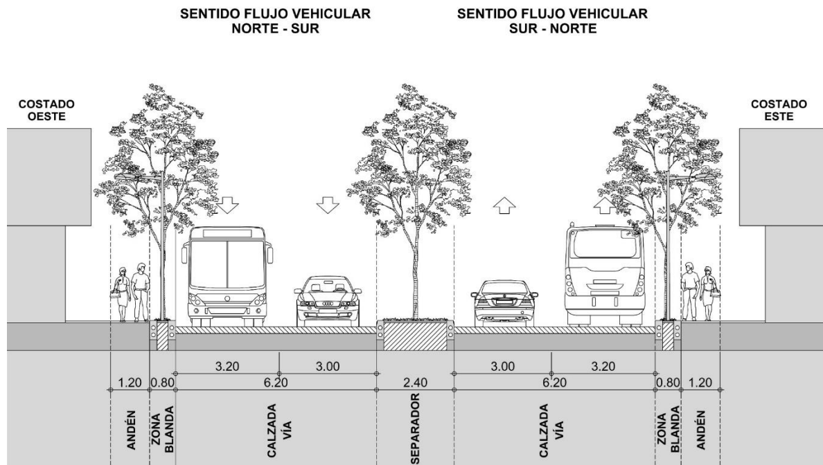
PERFIL TIPO CL 52 ENTRE KRA 8 Y KRA 26
