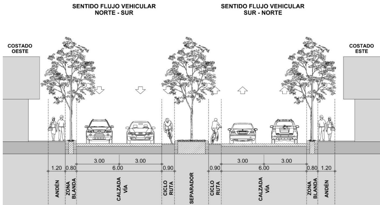
PERFIL TIPO CL 29 ENTRE KRA 29 Y KRA 40B
