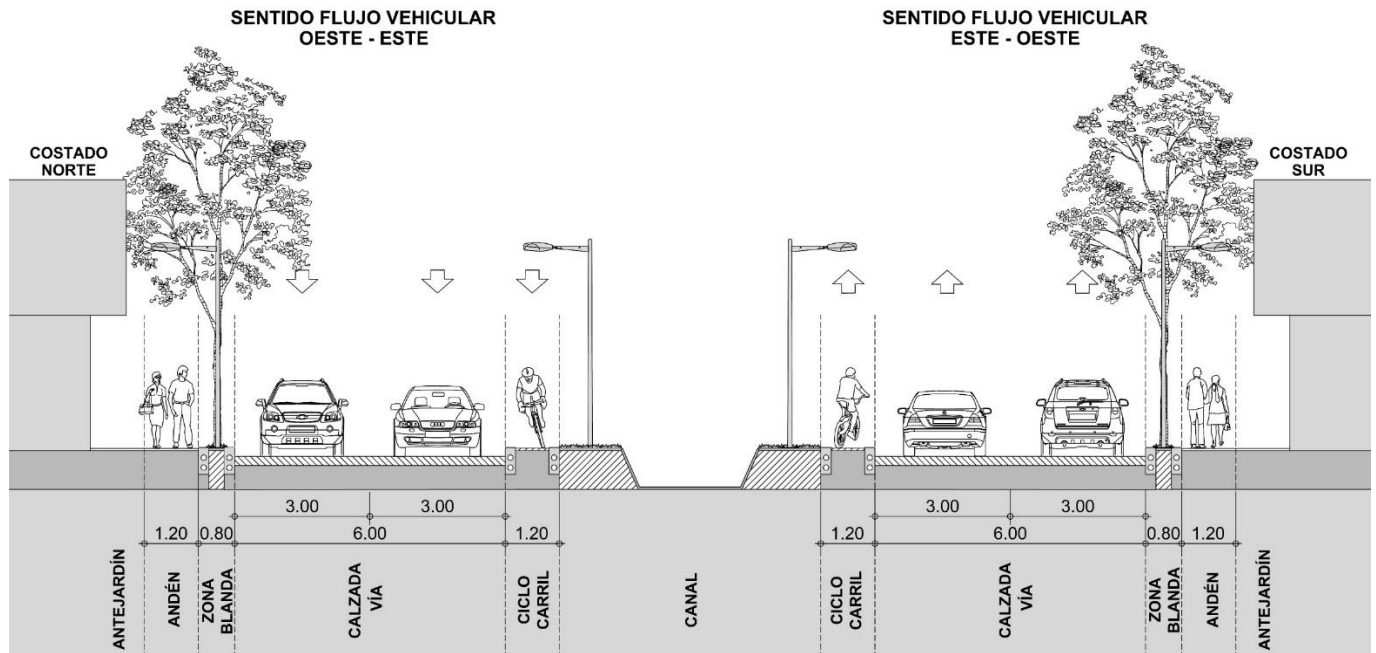
PERFIL TIPO KRA 27 ENTRE DG 28A Y DG 28C KRA 27 ENTRE CL 44 Y CL 70
