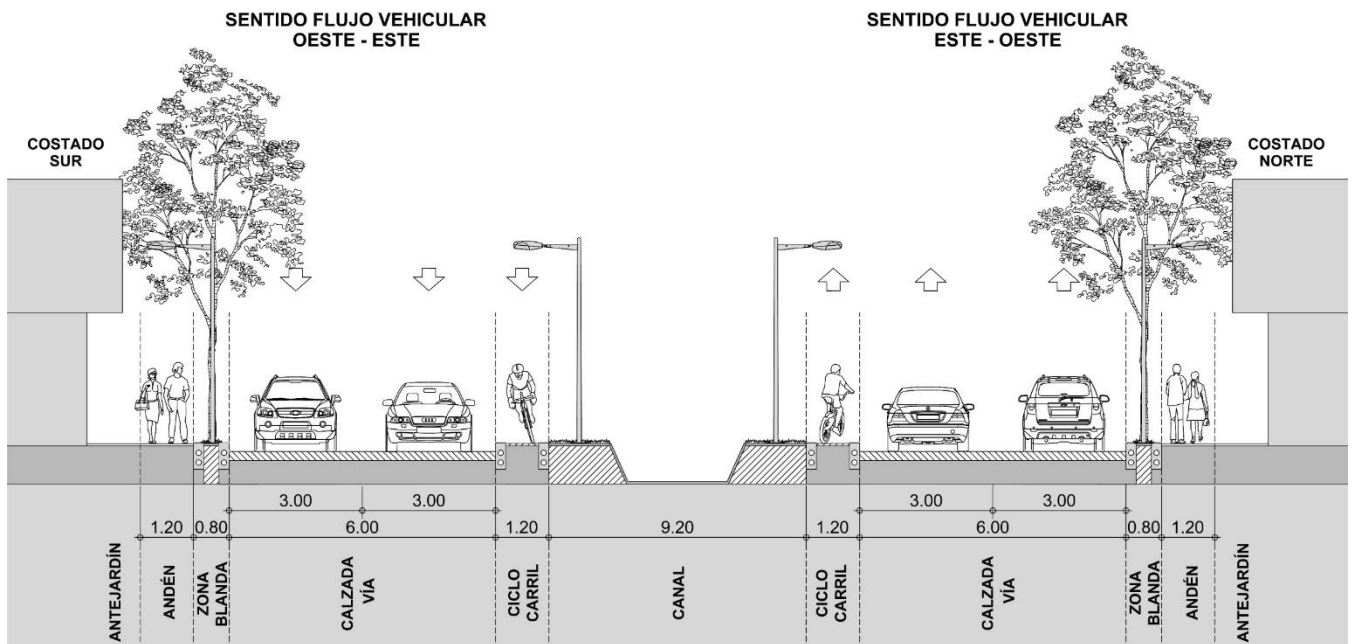
PERFIL TIPO KRA 28D ENTRE CL 44 Y CL 70
