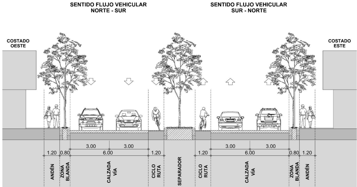
PERFIL TIPO KRA 25A ENTRE CL 33C Y CL 42 KRA 34 ENTRE CL 25 Y CL 35
