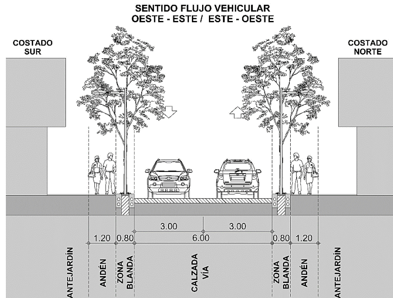
PERFIL TIPO KRA 17B ENTRE CL 33 F Y CL 40
