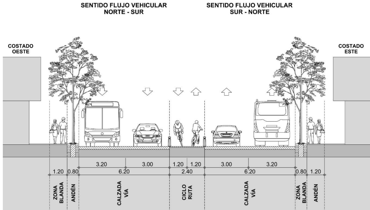
PERFIL TIPO CL 59 ENTRE KRA 8 Y KRA 15
