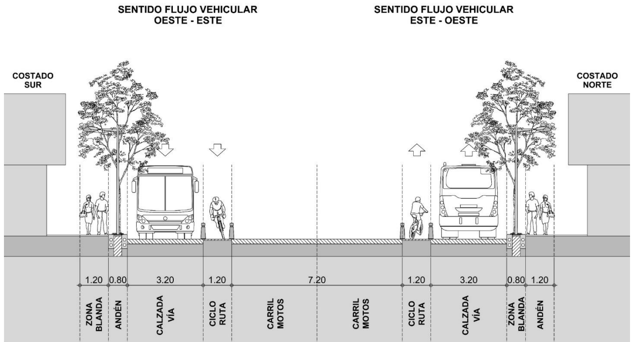
PERFIL TIPO KRA 27 ENTRE DG 28A Y DG 28C KRA 27 ENTRE CL 44 Y CL 70
