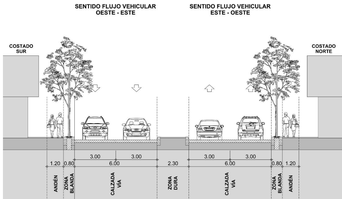
PERFIL TIPO KRA 40B ENTRE CL 27 Y CL 29
