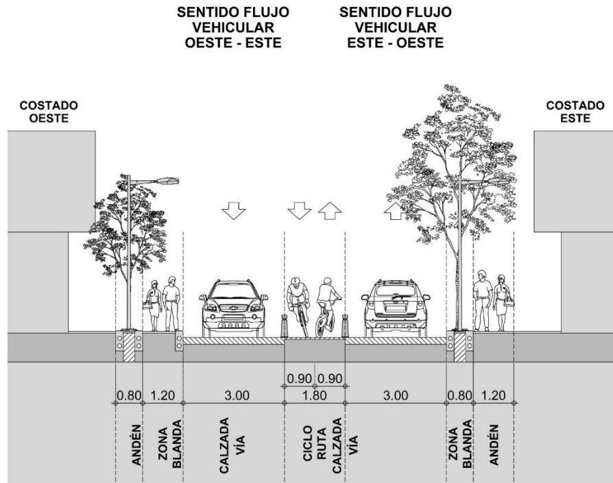
PERFIL TIPO CL 52 ENTRE KRA 8 Y KRA 26
