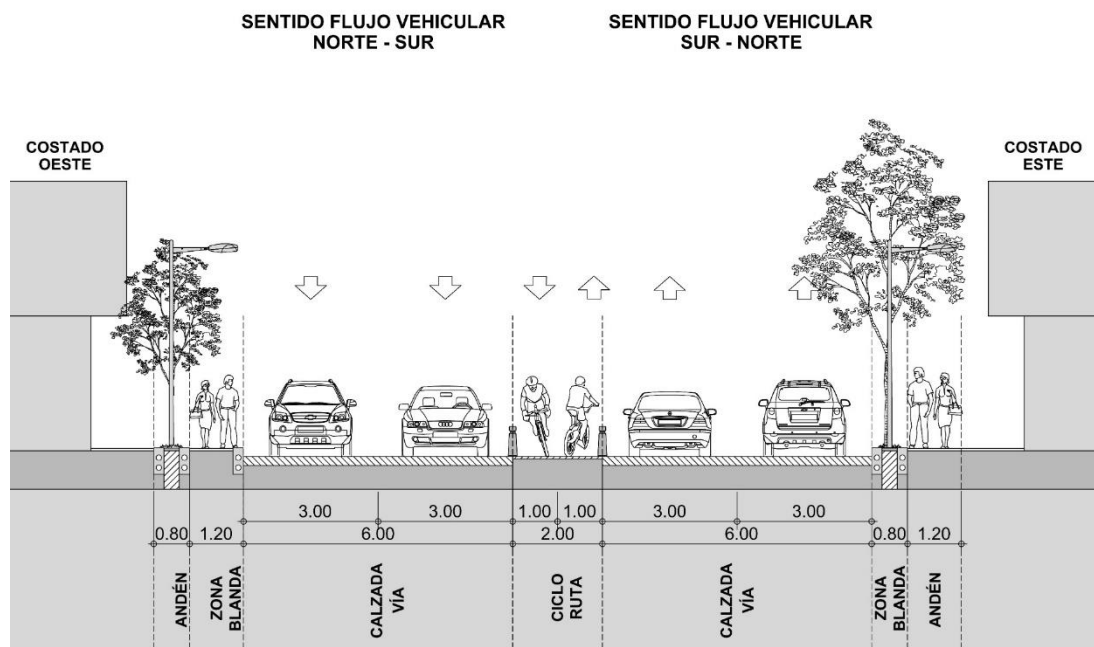
PERFIL TIPO CL 34 ENTRE KRA 8A Y KRA 23
