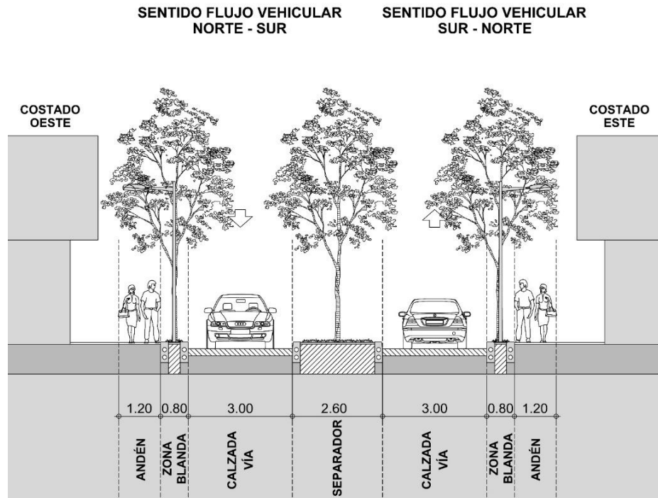
PERFIL TIPO CL 44 ENTRE KRA 28D Y KRA 32
