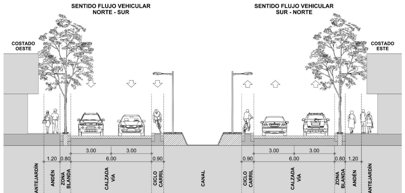
PERFIL TIPO CL 44 ENTRE KRA 28D Y KRA 32
