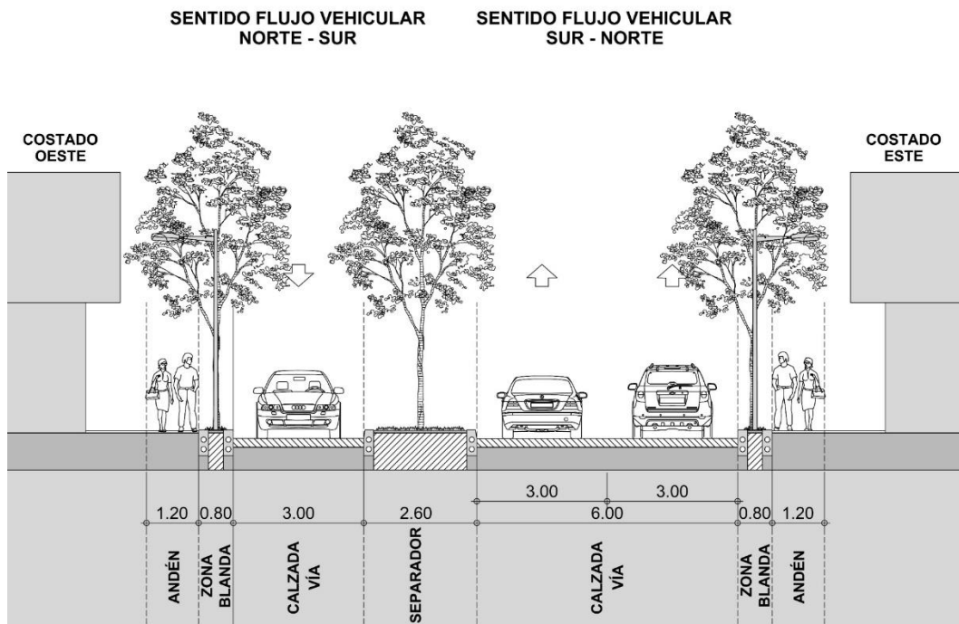
PERFIL TIPO CL 39 ENTRE KRA 25A Y KRA 26B
