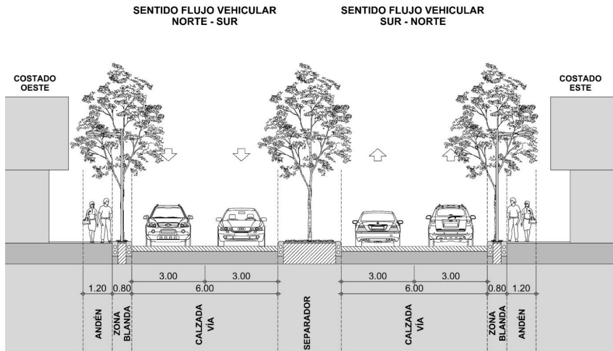
PERFIL TIPO CL 30A ENTRE KRA 41 Y DG 28C
