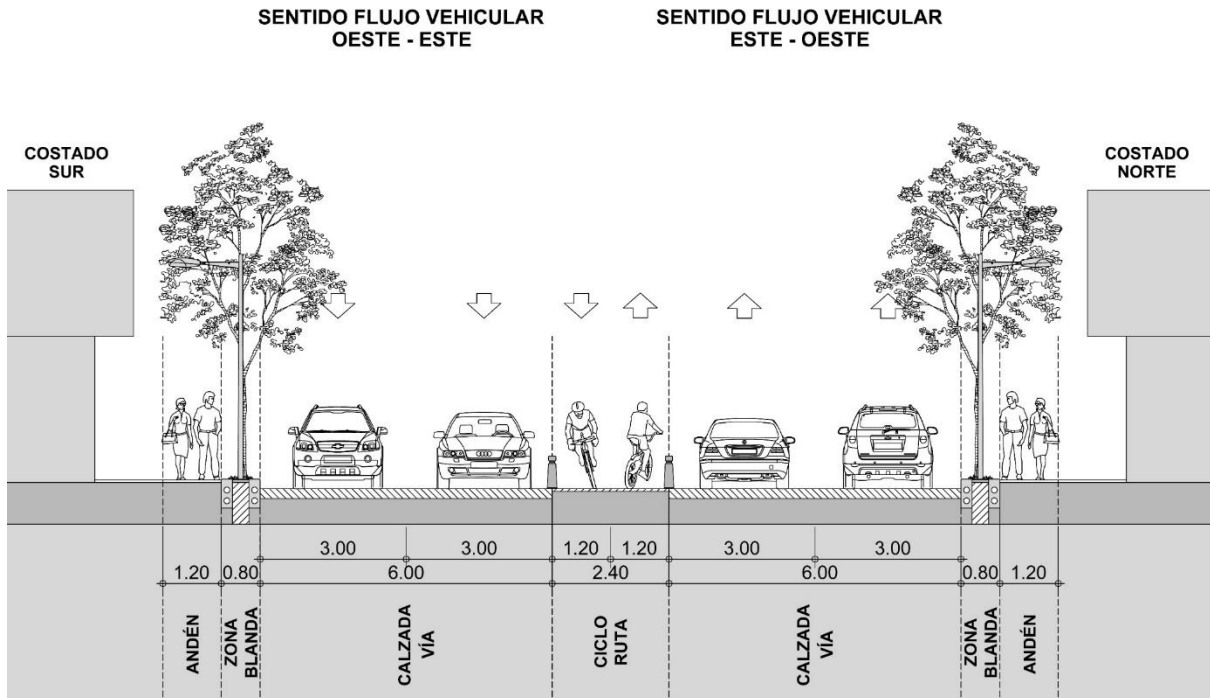
PERFIL TIPO KRA 28D ENTRE CL 44 Y CL 70
