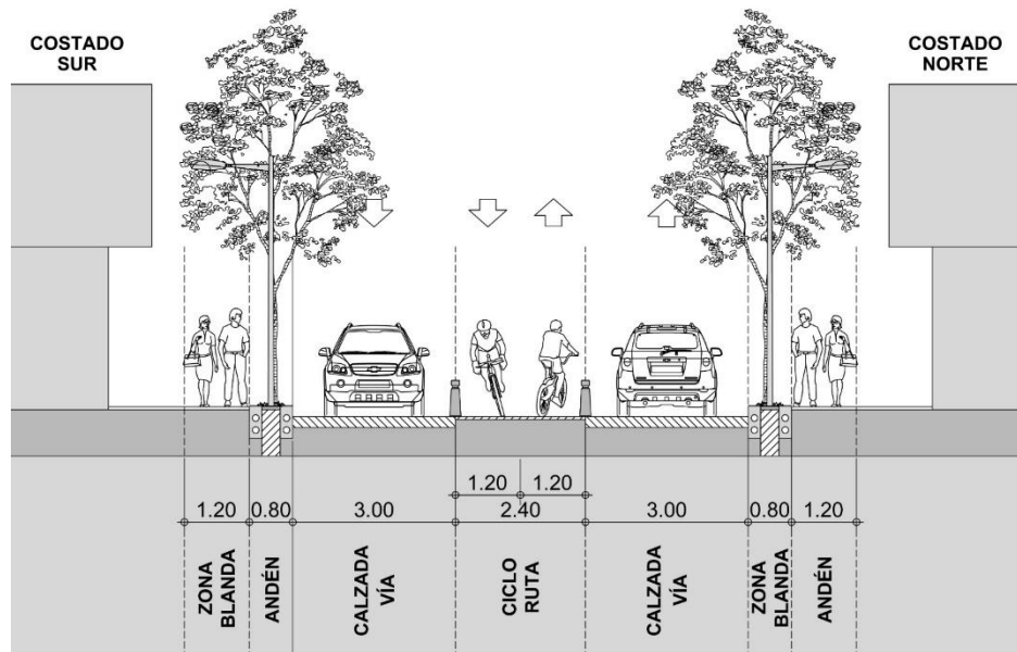
PERFIL TIPO KRA 12 ENTRE CL 39 Y CL 45
