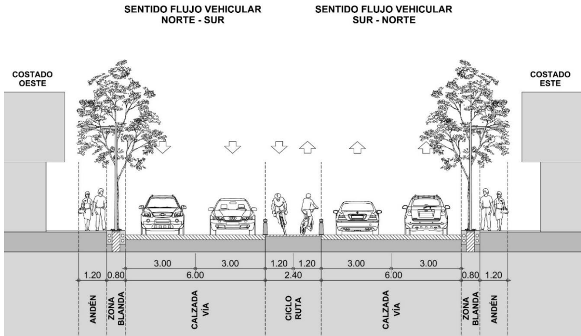
PERFIL TIPO CL 39 ENTRE KRA 25A Y KRA 26B
