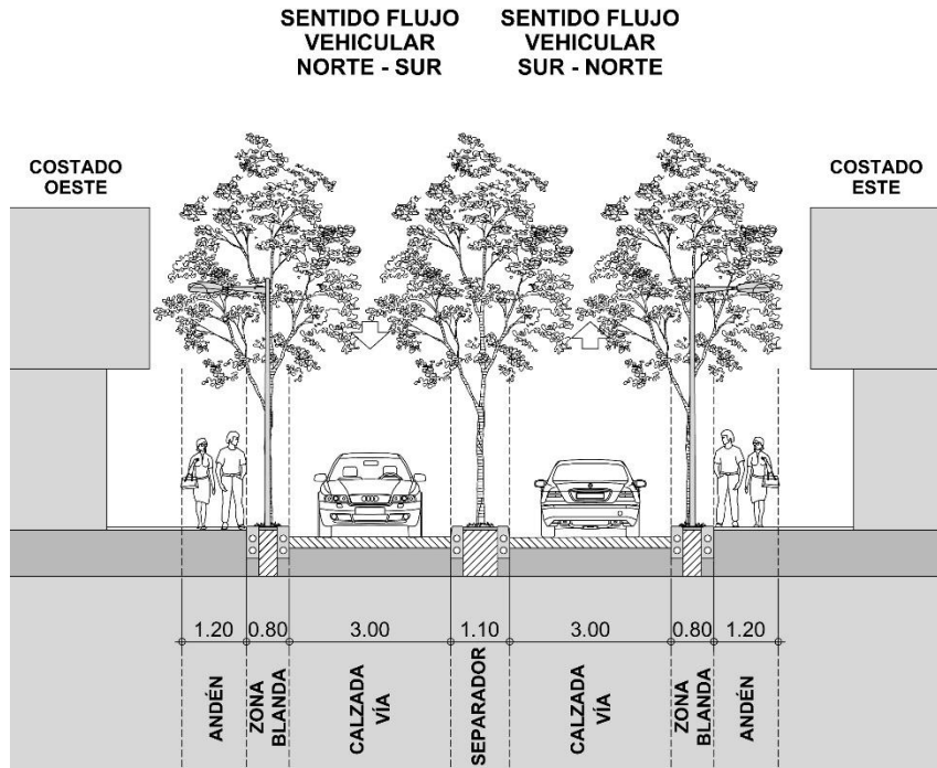
PERFIL TIPO CL 30A ENTRE KRA 41 Y DG 28C
